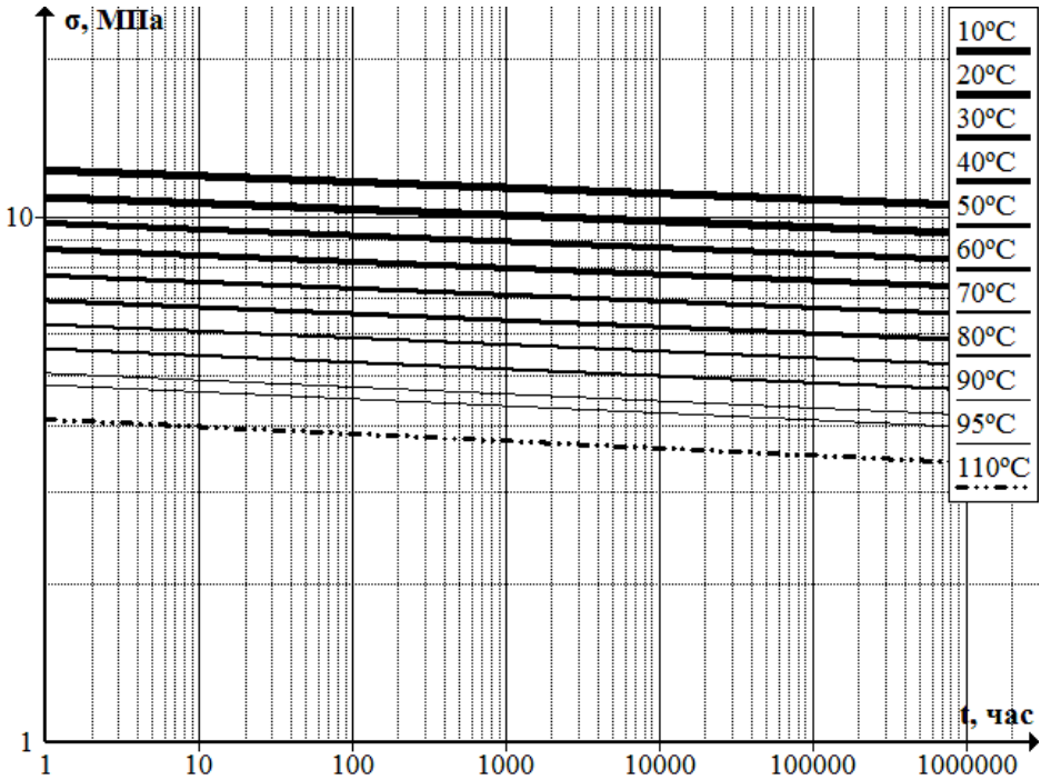
Рисунок 1 – Графики длительной прочности труб PRADEX PE-Xa при различных температурах теплоносителя ( \sigma – кольцевые напряжения; t – время работы до разрушения трубы)
